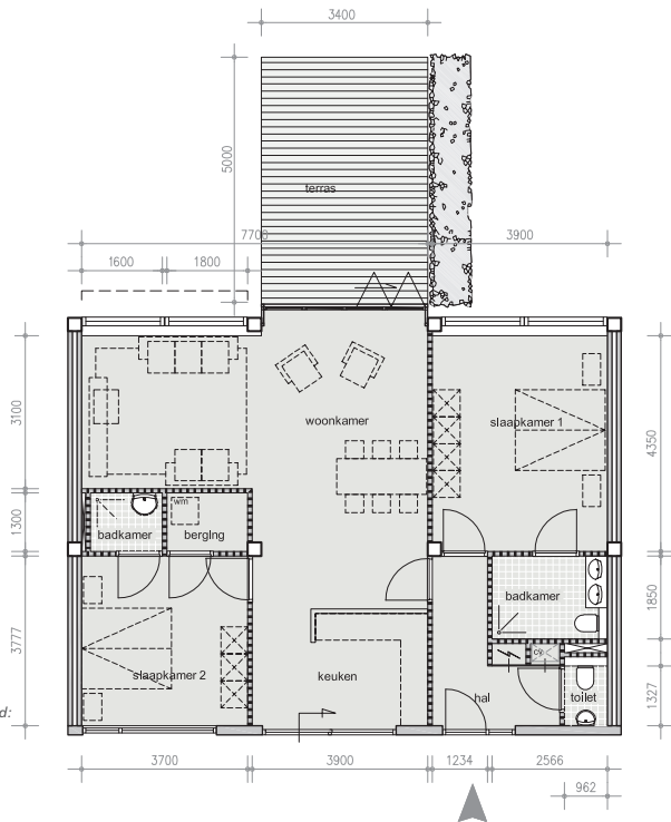
Bouwnummer 51 verdieping
